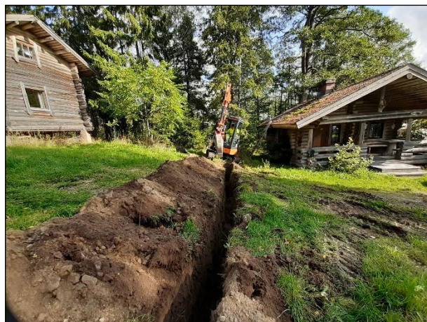
Vasen: maaperä pihan alueella oli hiekkaa, seassa oli joitakin suuria kiviä. Oikea: kaapeloja kaivettiin kahden piharakennuksen välistä, alueella oli aikaisempi kaapelikaivanto rakennusten välillä.
